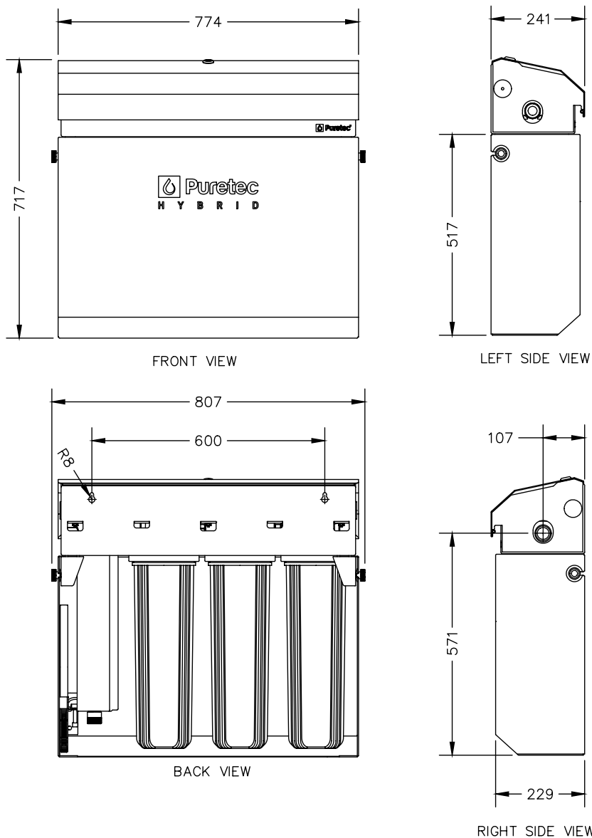
Fig. 5 - E13AMC Dimensions
